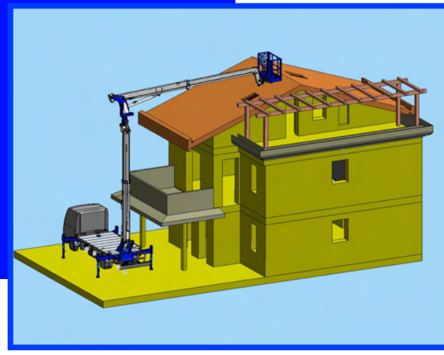
Ottima altezza di scavalco ostacoli, scavalco "pulito" in quanto i bracci inferiori sono verticali "modalità di lavoro 2" Excellent overcoming-obstacles height - Third configuration
