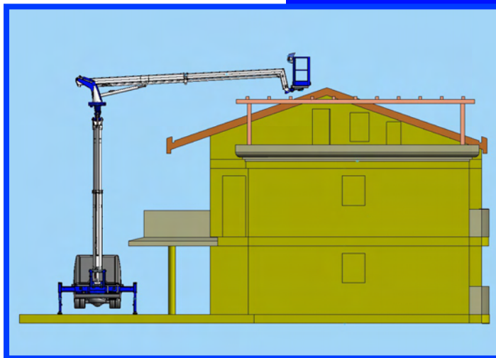
Ottima altezza di scavalco ostacoli, scavalco "pulito" in quanto i bracci inferiori sono verticali "modalità di lavoro 2" Excellent overcoming-obstacles height - Third configuration
