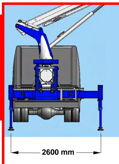
Ingombro negativo nullo in tutte le configurazioni. Stabilizzazione HE, possibilità di estendere solo da una parte con un ingombro di 2600 mm Zero Tailswing in all the configurations. Working area with stabilizers straight down - Working area with stabilizers hydraulically extendible "One side" working area
