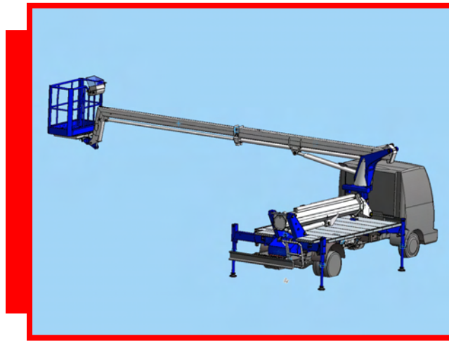
Possibilità di lavorare come semplice telescopica "modalità di lavoro 1" Possibility of working as pure telescopic - Second configuration
