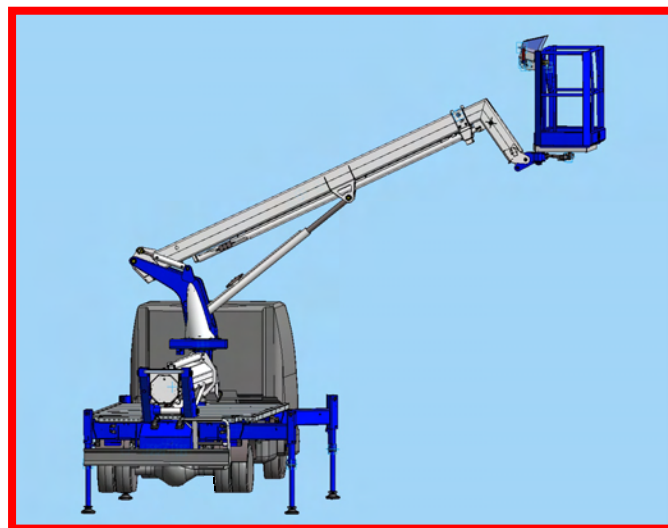
Ingombro negativo nullo in tutte le configurazioni. Stabilizzazione HE, possibilità di estendere solo da una parte con un ingombro di 2600 mm Zero Tailswing in all the configurations. Working area with stabilizers straight down - Working area with stabilizers hydraulically extendible "One side" working area
